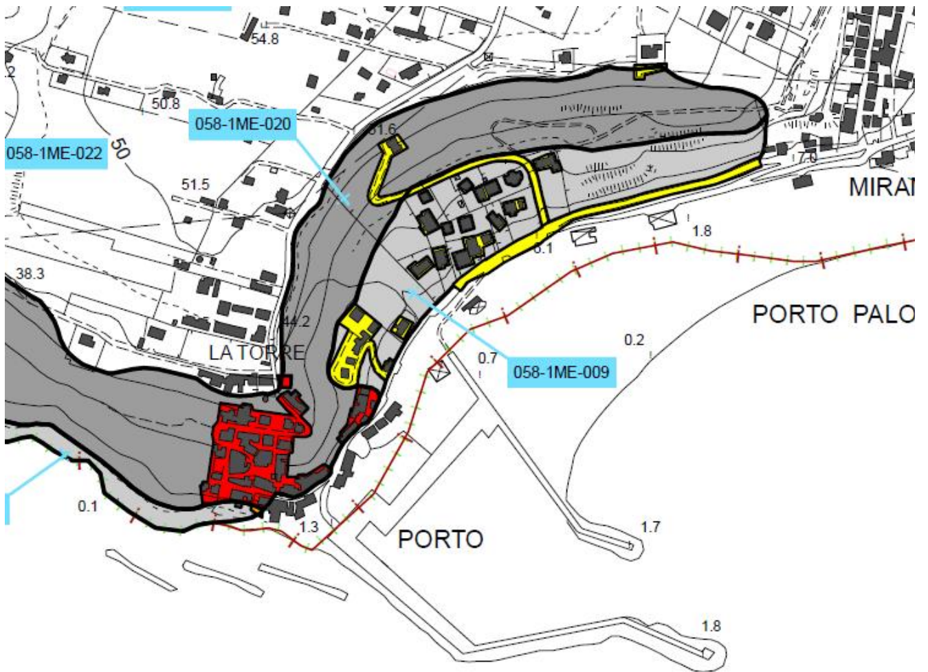
Stralcio del Piano di Assetto Idrogeologico
